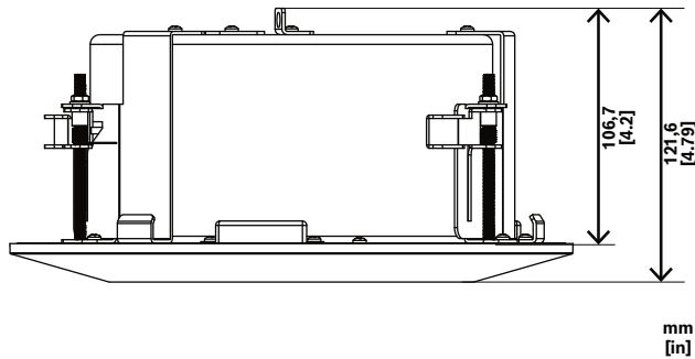
Abb. 2: NDA-8002-PLN Nicht-IR Abmessungen in mm (Zoll)
