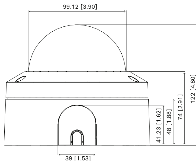
Abmessungen in mm (Zoll)
