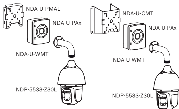
Abb. 2: Masthalterung (IP66), Eckhalterung (IP66)
